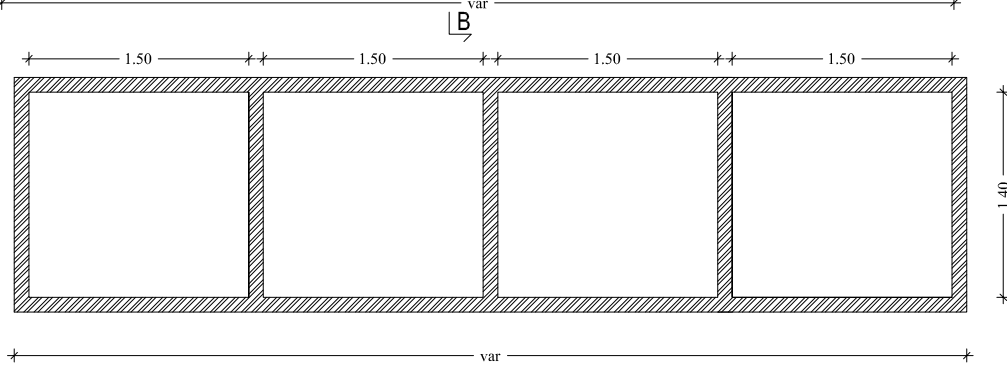
VISTA FRONTALE A-A
